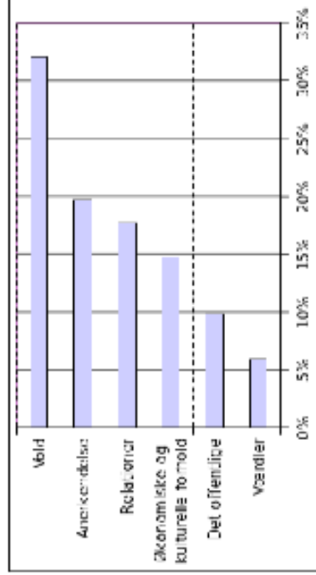
Figur 1: Årsagernes forklaringsandele
